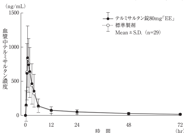
80mg錠1錠投与時の平均血漿中薬物濃度推移
